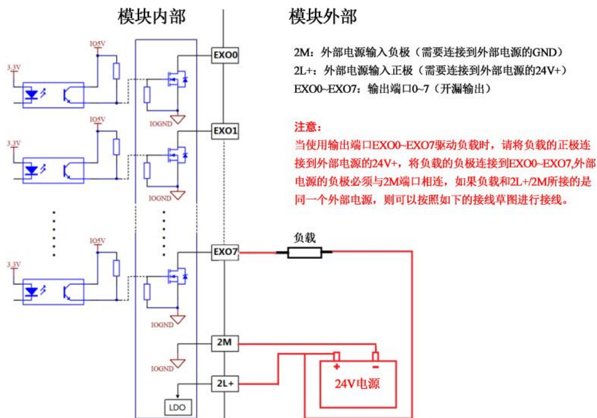
图 2-8 6 轴模块输出部分接线说明
