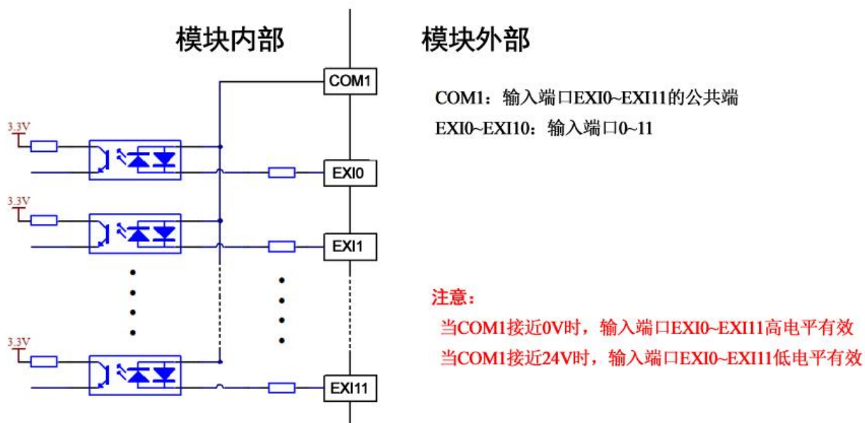
图 2-9 6 轴模块输入部分接线说明
