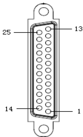
图 2-4 AXIS1~AXIS6 接口
