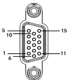
图 2-5 MPG 接口示意图
