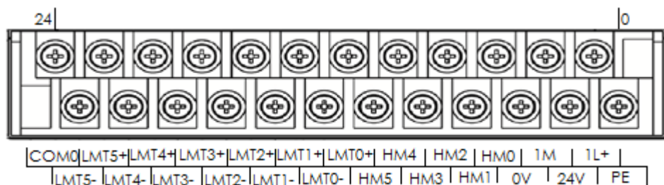
图 2-2 电源、限位及 HOME 输入接口
