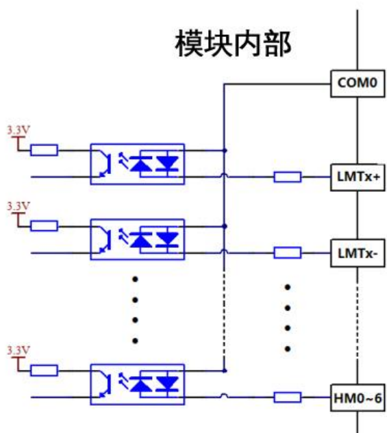
图 2-7 6 轴模块输入部分接线图
