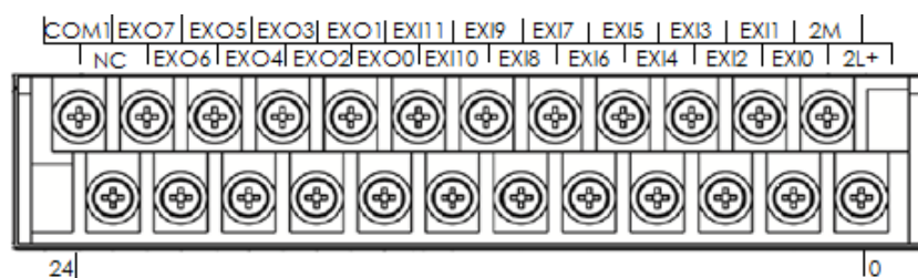
图 2-3 电源、通用 I/O 接口
