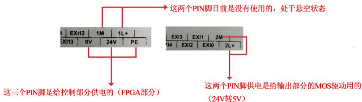
图 2-10 6 轴模块外壳丝印说明（供电引脚说明）
